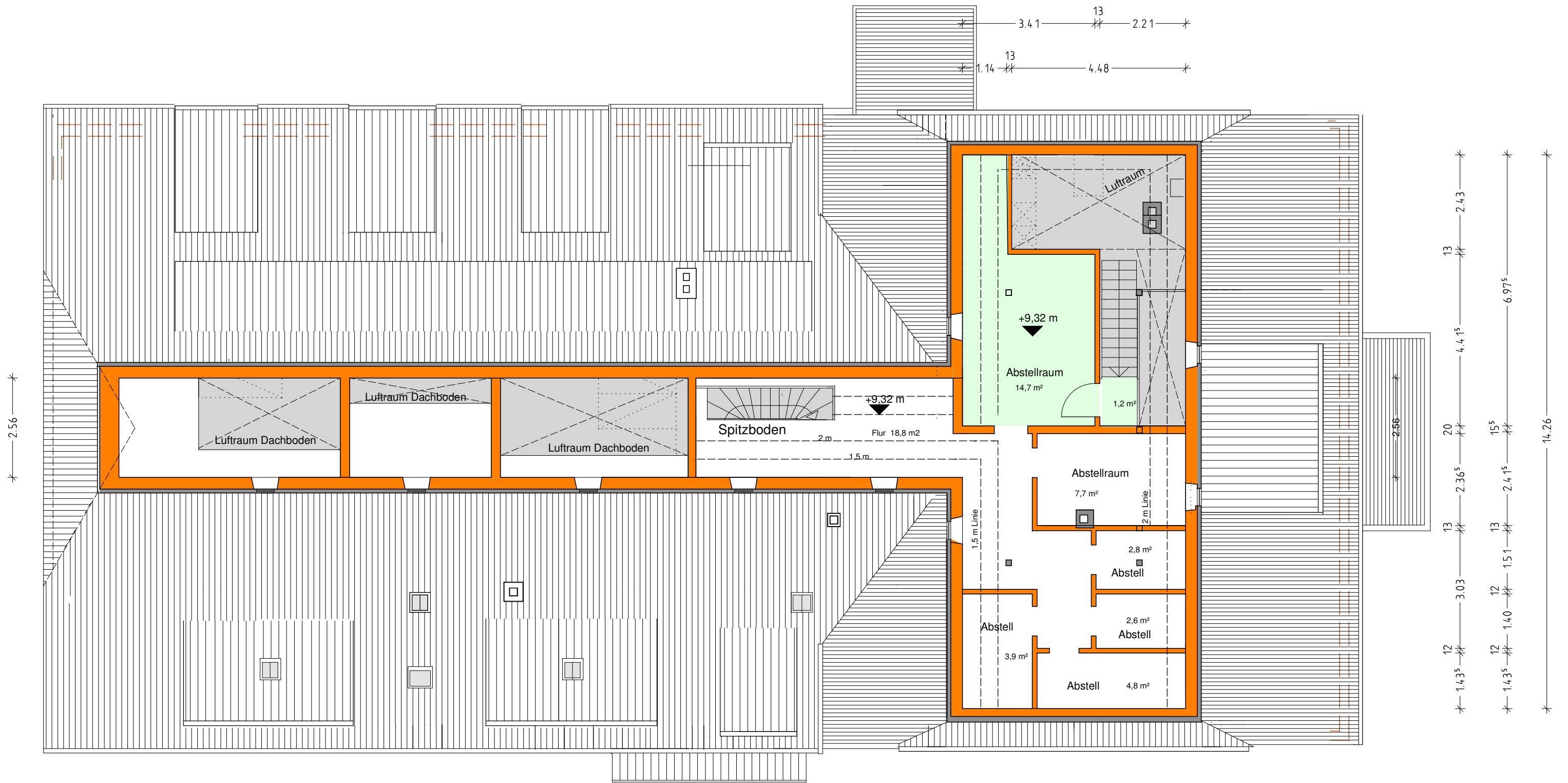
GRUNDRISS DACHBODEN VARIANTE 12
