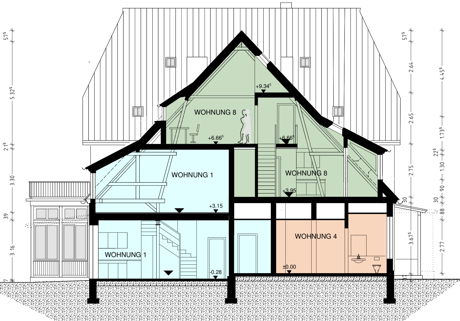
SCHNITT A-A 12
