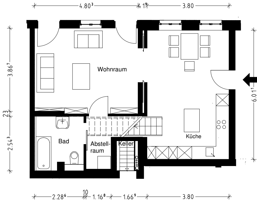
GRUNDRISS ERDGESCHOSS
